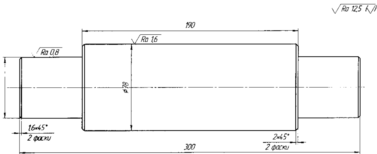
Рисунок 1– Деталь-вал.
